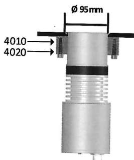
HMHT01/HMHT-EX01
